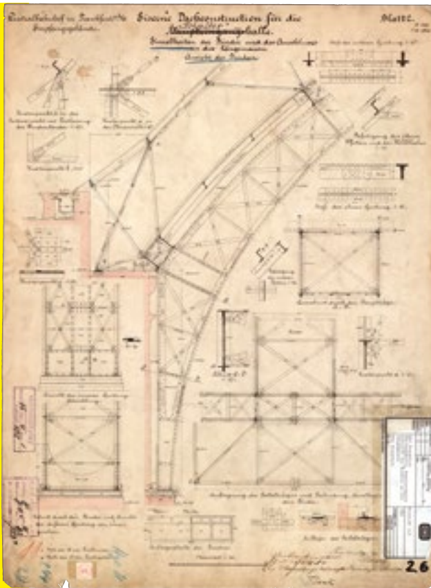
Dachkonstruktion für die Schaltheralle des Hauptbahnhofes in Frankfurt, 1886 (HHStAW Abt. 3011/1 Nr. 10830 V)
