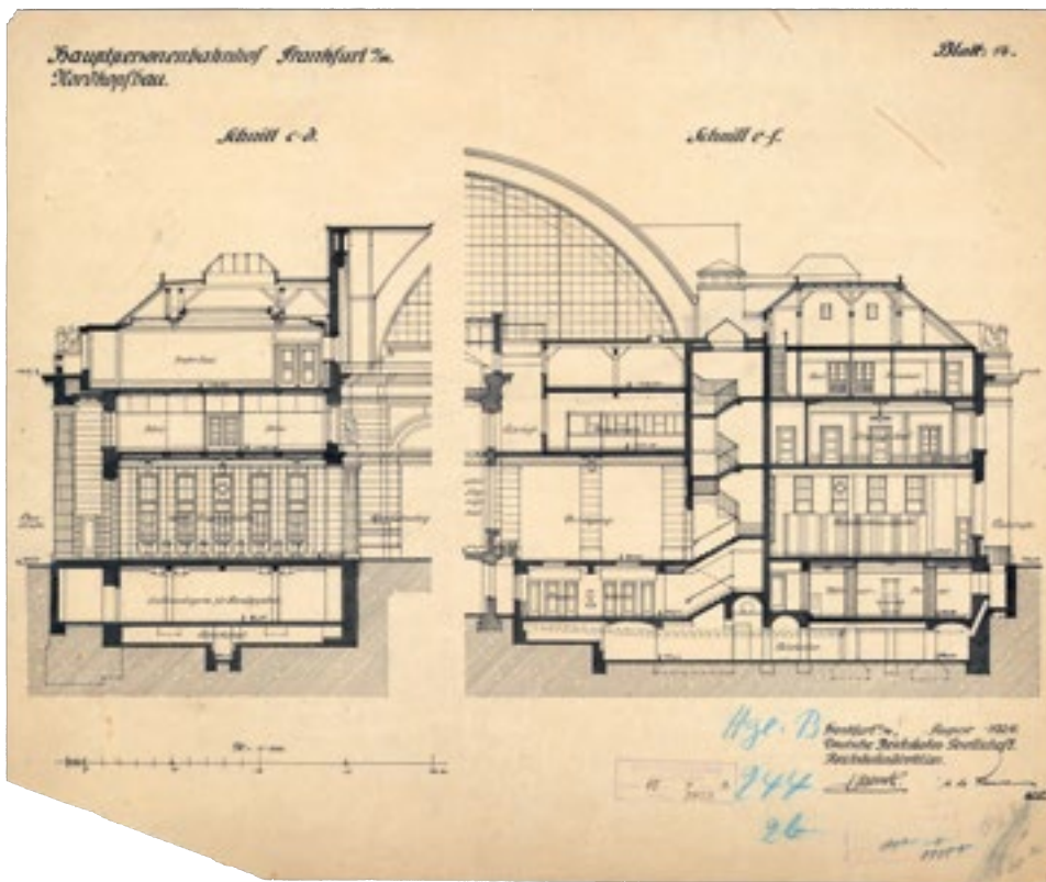
Erweiterung des Empfangsgebäudes des Hauptbahnhofs in Frankfurt, Nordflügel (Ansicht), 1913 (HHStAW Abt. 3011/1 Nr. 10833 V)
